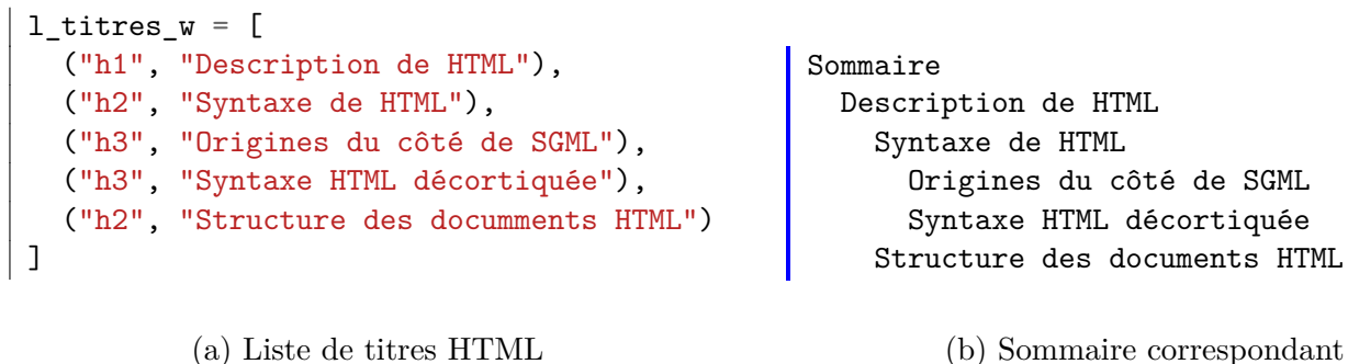
FIGURE 9 – Entrée et sortie de notre production de sommaire.
