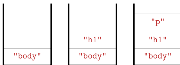
FIGURE 7 – Étapes de l'algorithme sur codeHTML3 , la valeur renvoyée à la fin est False .
